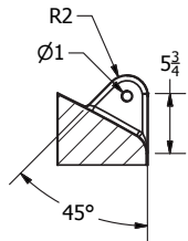
SECTION A-A SCALE 1:12
